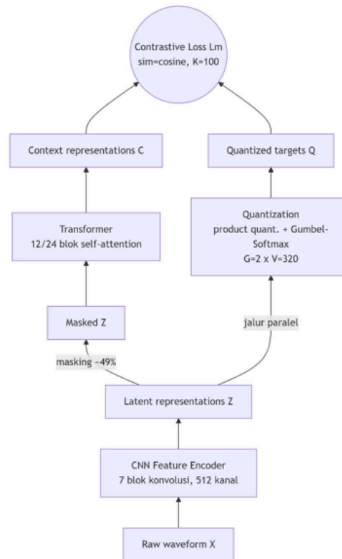
Gambar 2.1 Arsitektur Wav2vec2
