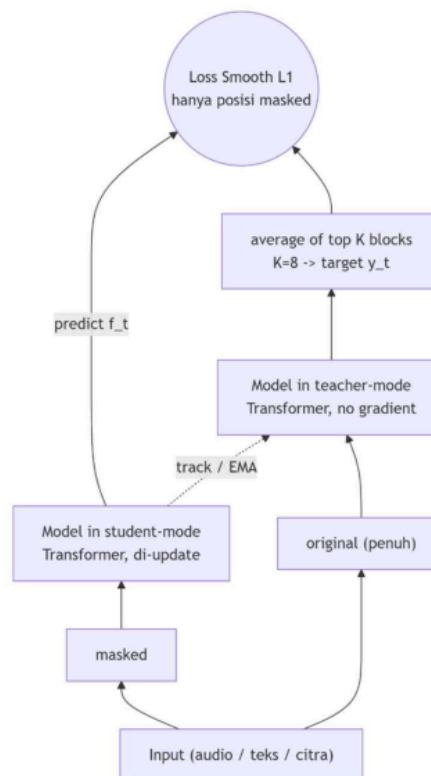
Gambar 2.2 Arsitektur Data2vec
