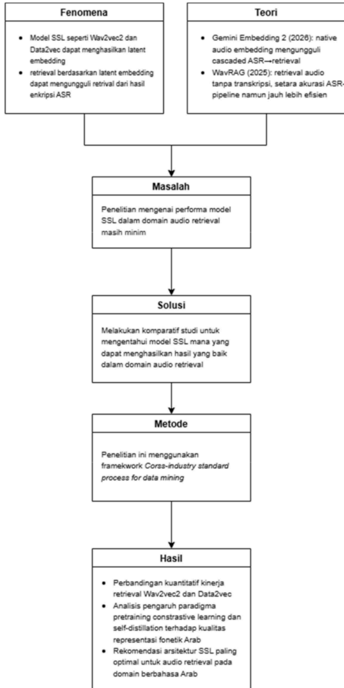
Gambar 1.1 Kerangka Pemikiran
